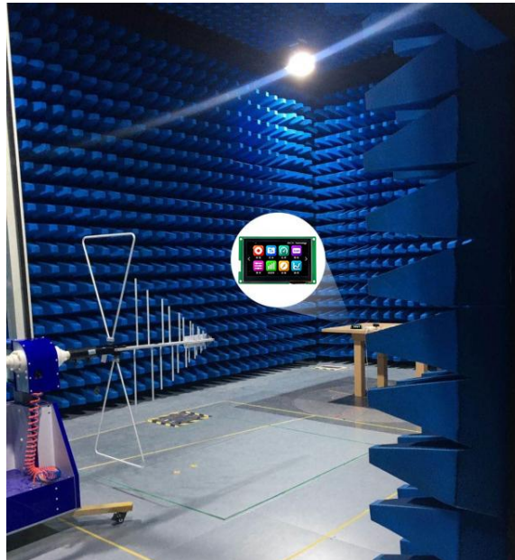
图 4-4 RE 测试图
