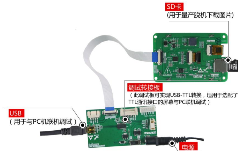
图 1-3 调试工具图
