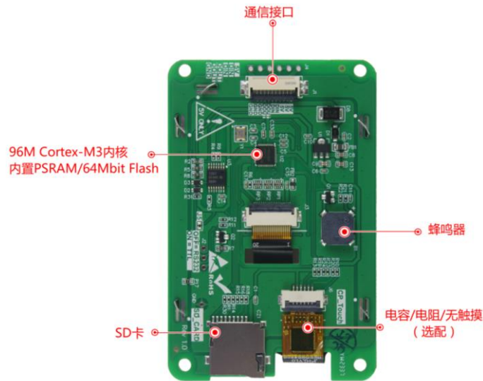
图 1-2 硬件配置图
